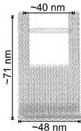
Schematische Darstellung der DNA-Origami-Nano-Antenne mit Abmaßen in Nanometer
