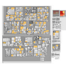
EvoCells Treemap
