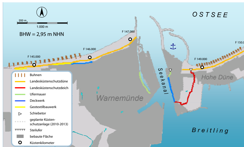
Abbildung 2.6: Sturmflutschutzsystem Warnemünde, Quelle: „Regelwerk Küstenschutz Meckenburg-Vorpommern“, 2009.
