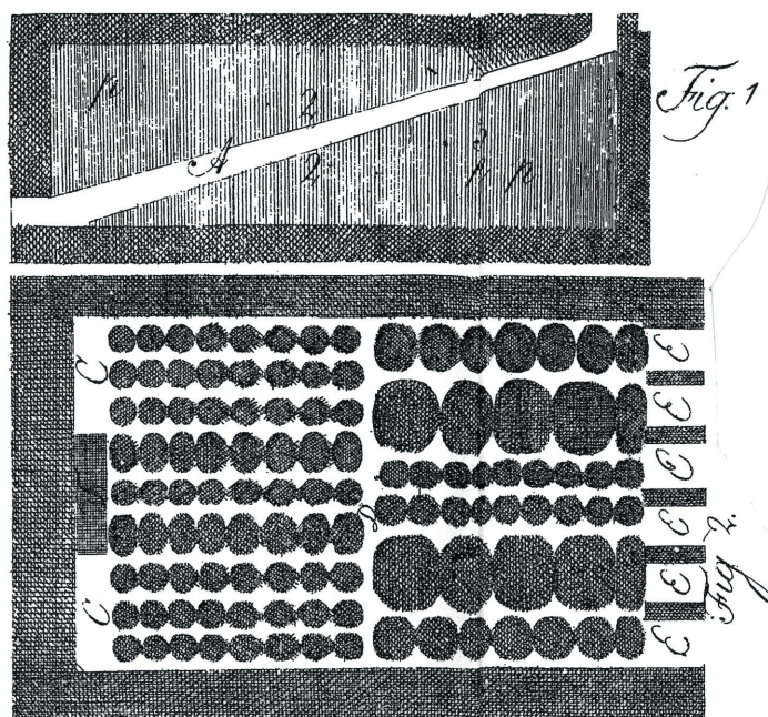
Abb. 2: Skizze eines Wiener Ofens. Quelle: Weber 1798, Tafel VI, Fig. 1 und 2
