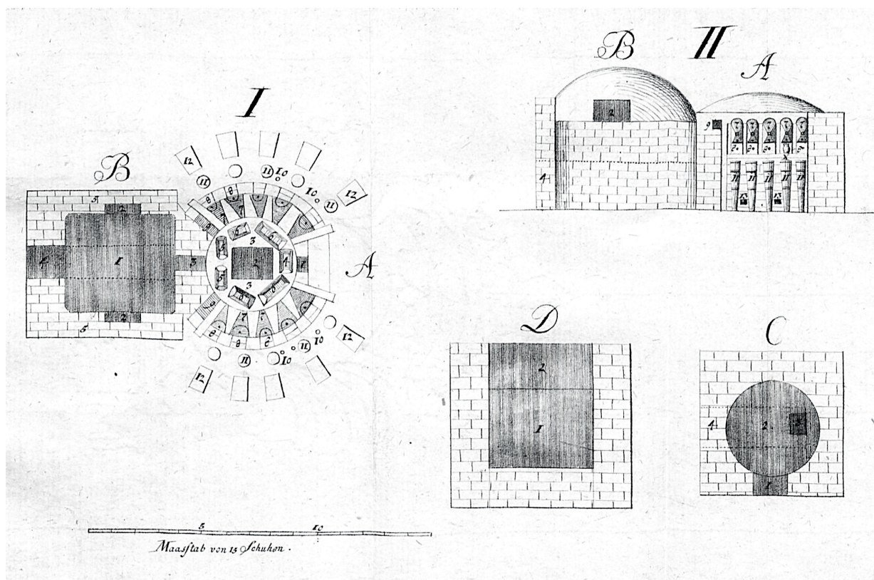
Abb. 5: Skizze einer Glasschmelzanlage für die Herstellung von Glasknöpfen und Glasperlen in Warmensteinach aus dem Jahr 1791; A) Glasschmelzofen, B) Asch- und Einbrennofen, C) Aufwärmofen und D) Holzdörrofen. Quelle: Forschungsbibliothek Gotha der Universität Erfurt, Geogr 8° 2378/2, Flurl 1792, Tafel III
