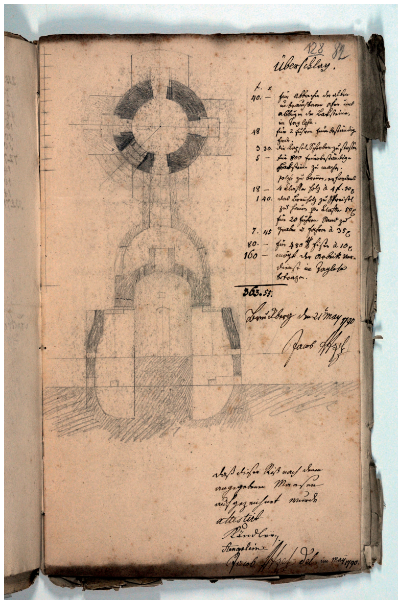
Abb. 3: Skizze eines zweietagigen Rundofens für die Porzellanmanufaktur Bruckberg, angefertigt von Johann Eberhard Stengelein im Jahr 1790. Quelle: Stiftung Preußische Schlösser und Gärten Berlin-Brandenburg, KPM-Archiv, Sign. 294, Bl. 128 bzw. 82
