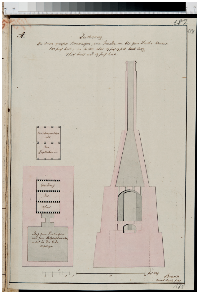
Abb. 1: Skizze für die Steingutbrennöfen in Rheinsberg, angefertigt von Bernhard Matthias Brasch im Jahr 1787. Quelle: Berlin, Geheimes Staatsarchiv Preußischer Kulturbesitz; II. HA, Gen. Dir., Fabr. Dpt., Abt. 25, Tit. 419, Nr. 30, Bd. 1, Bl. 189; Scan: GStA
