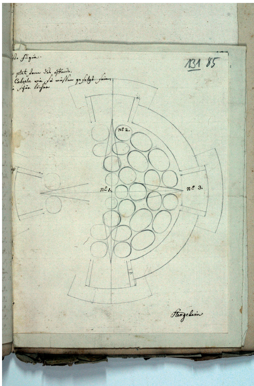
Abb. 8: Setzschem der Kapseln im zweietagigen Rundofen der Porzellanmanufaktur Bruckberg, gezeichnet von Johann Eberhard Stengelein. Quelle: Stiftung Preussische Schlösser und Gärten Berlin-Brandenburg; KPM-Archiv, Sign. 294, Bl. 131 bzw. 85
