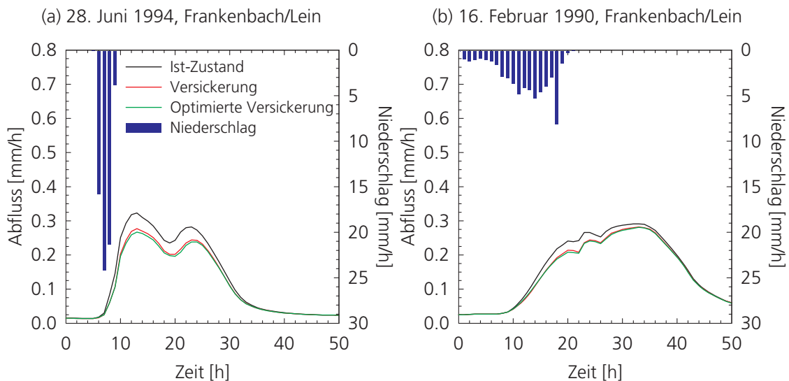
Abb. 5.27 Simulation zweier etwa 3-jährlicher Hochwasserereignisse im Einzugsgebiet der Lein für den Ist-Zustand und zwei Szenarien zur Niederschlagsversickerung in Siedlungsgebieten bei Anschluss von 1,3% der Einzugsgebietsfläche
