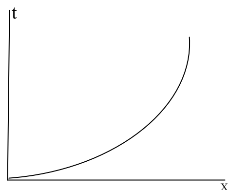
Direkte Progression
